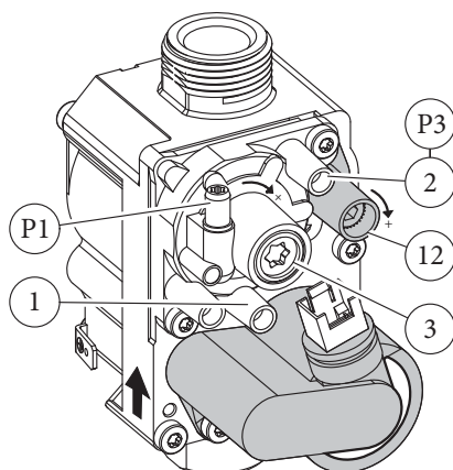
Plynový ventil 8205
