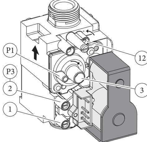
Plynový ventil 848
